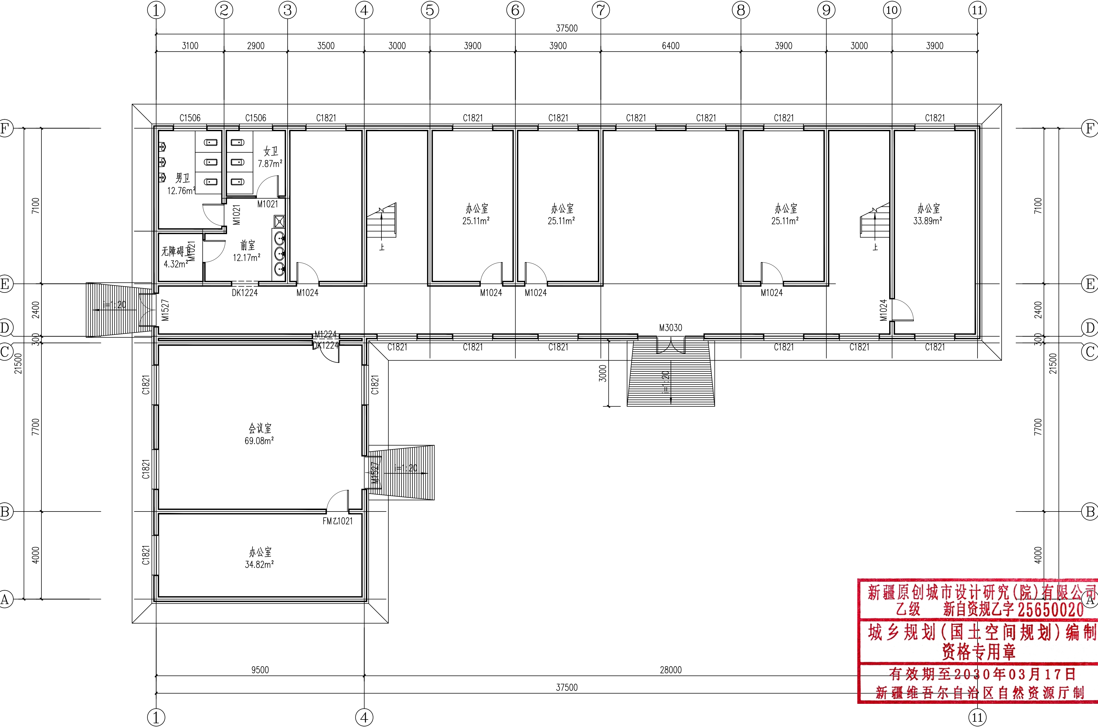
一层平面布置图 1:100
