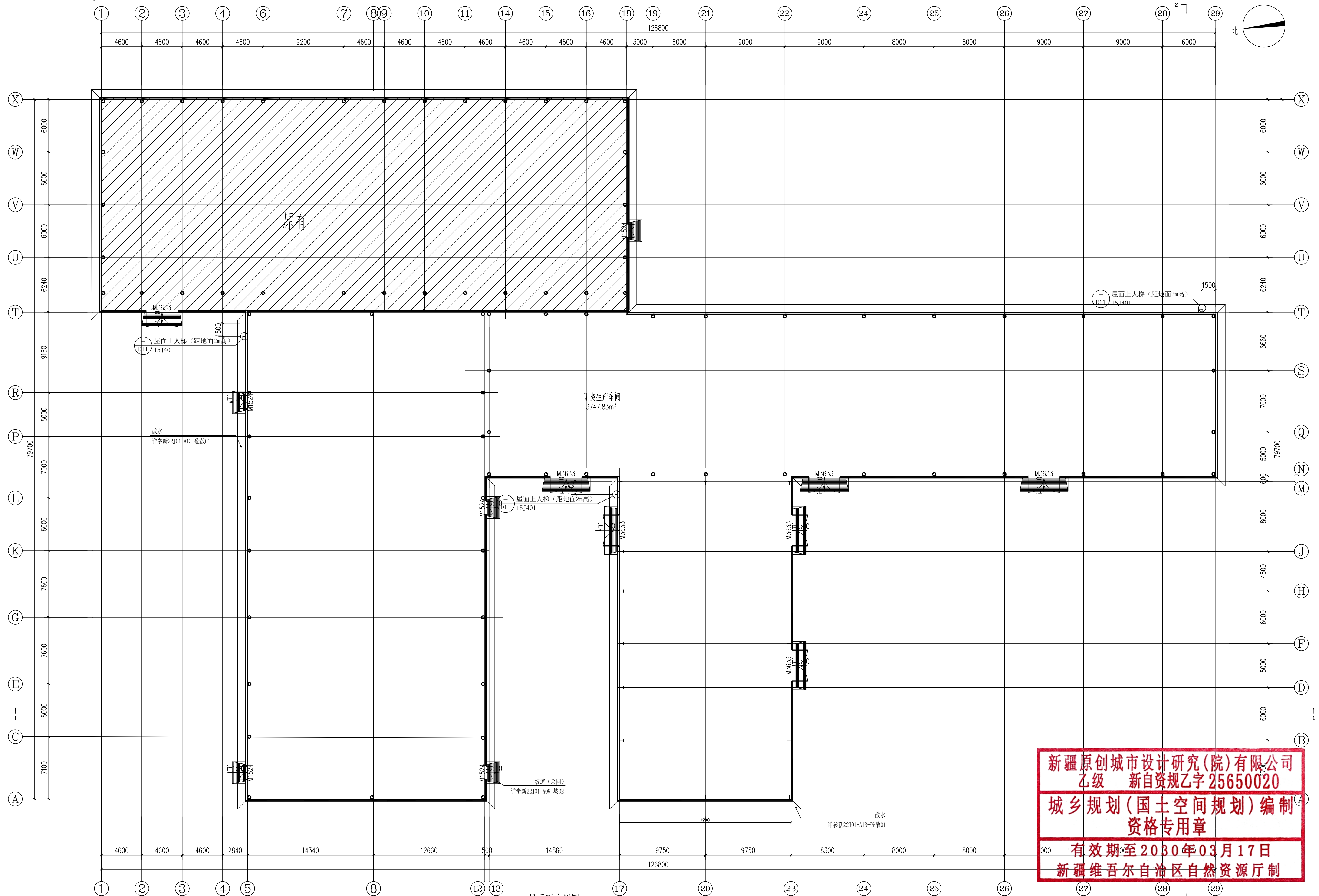
一层平面布置图 1:100
