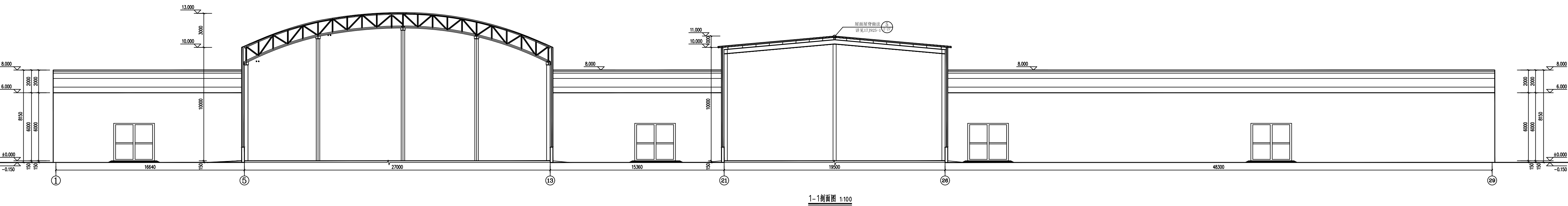
1-1剖面图 1:100
