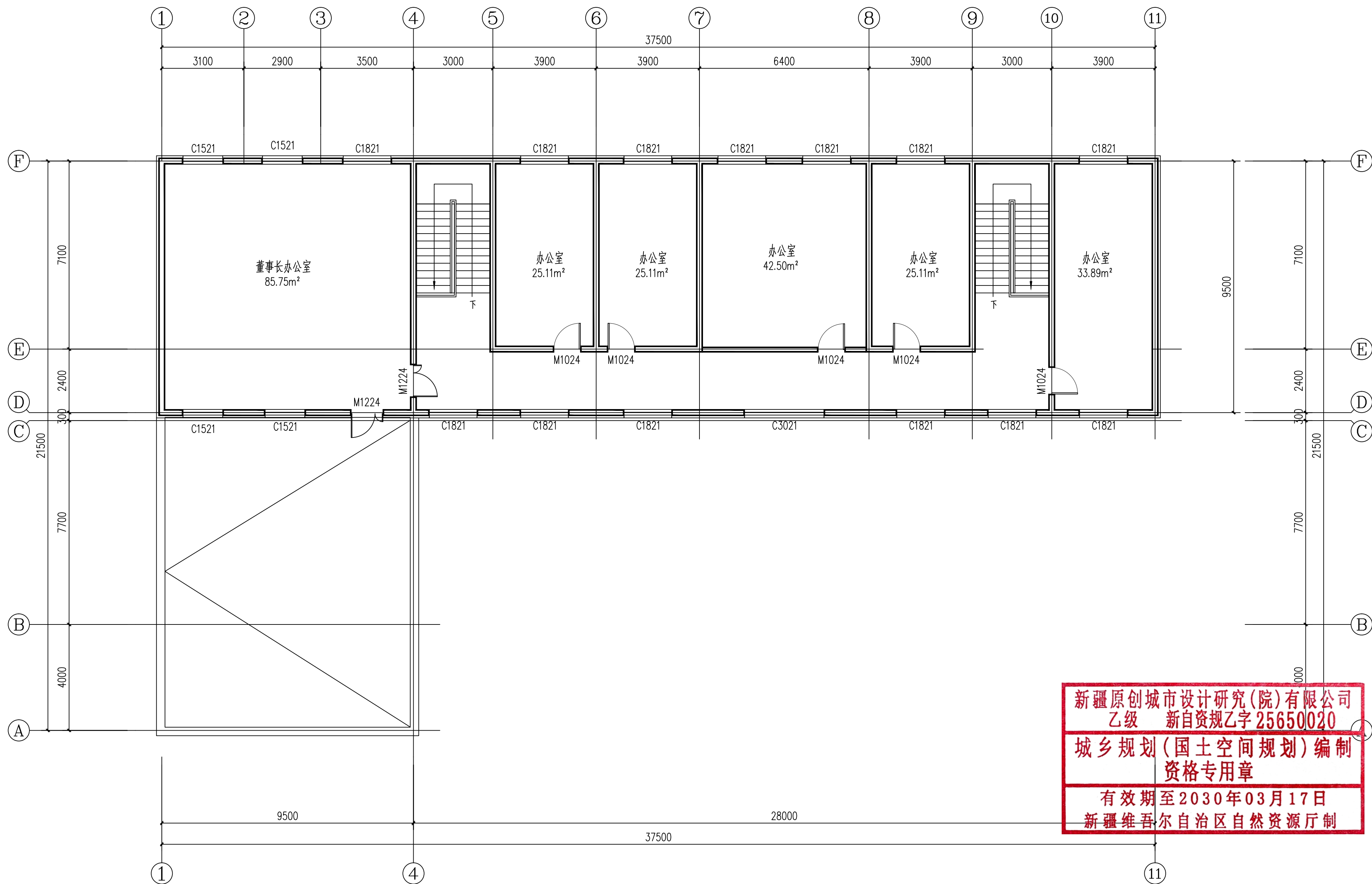
二层平面布置图 1:100
